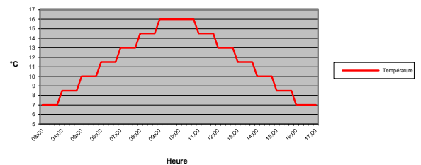
Evolution de la température avec la régulation MTP II
